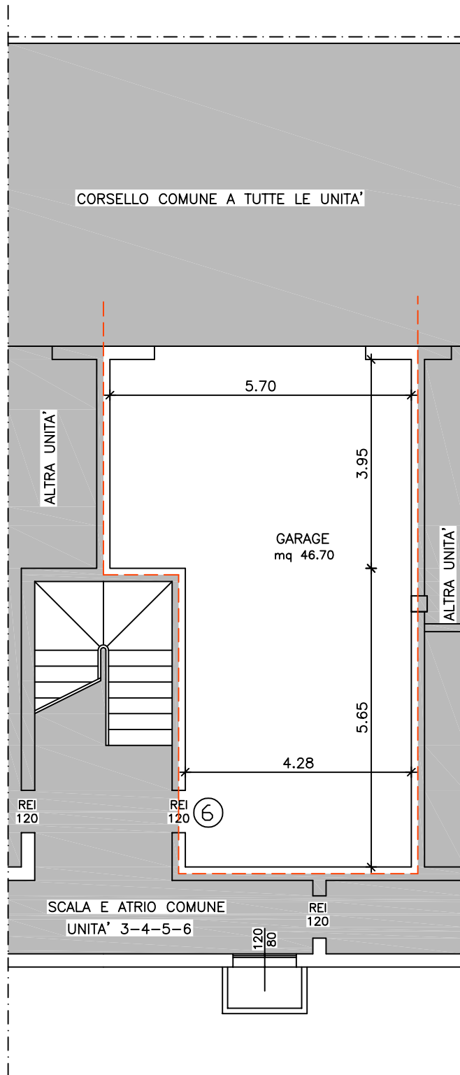
PIANTA PIANO INTERRATO SCALA 1:100
